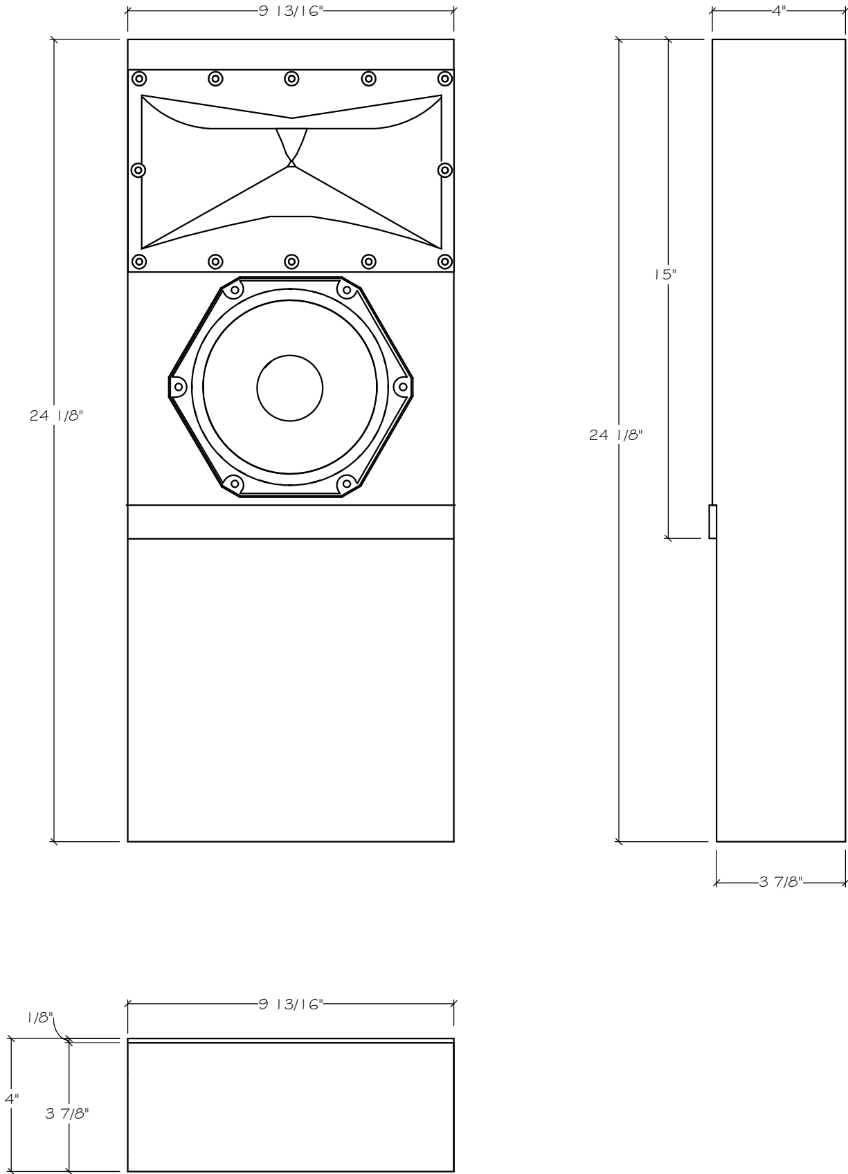
Rixos-SNR - Dimension Drawings
